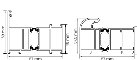
PROFIL NAŚWIETLA PROFIL OŚCIEŻNICY ALU/75
