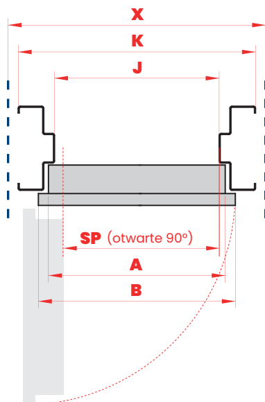
PRZEKRÓJ POZIOMY
