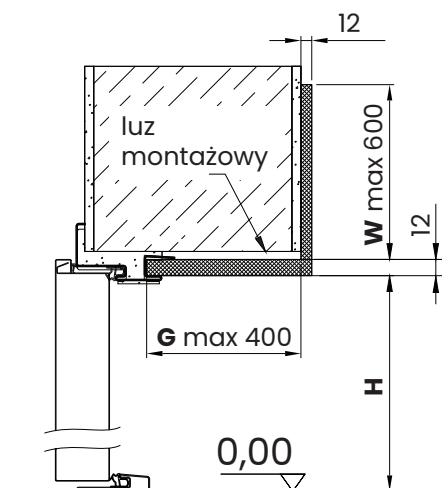
PRZEKRÓJ PIONOWY
