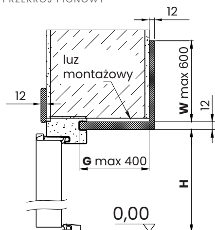
PRZEKRÓJ PIONOWY
