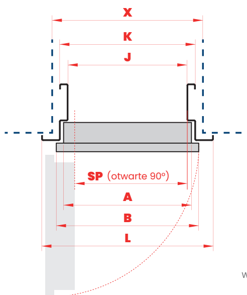
PRZĘKÓJ POZIOMY
