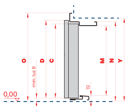
PRZĘKÓJ PIONOWY
