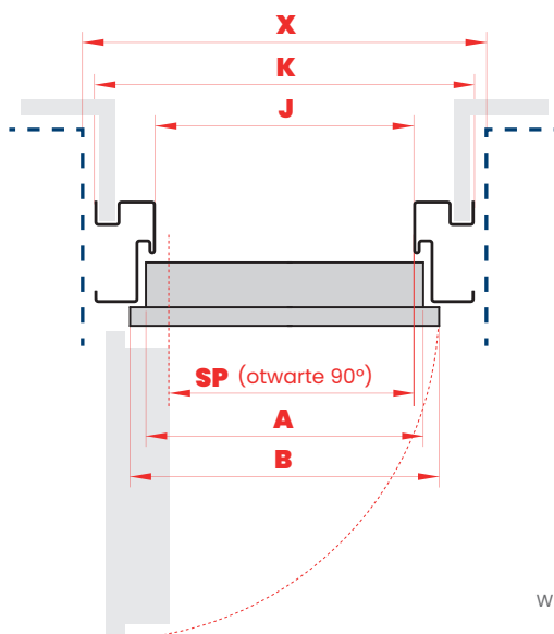
PRZEKRÓJ POZIOMY
