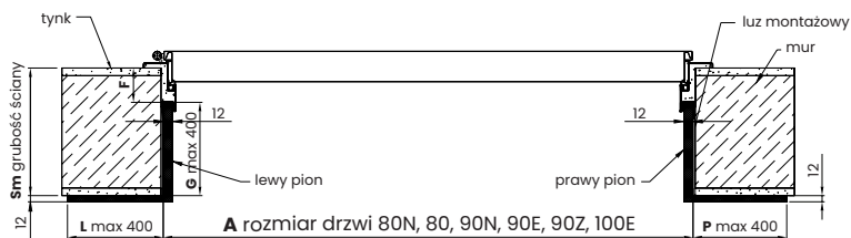
PRZEKRÓJ POZIOMY
