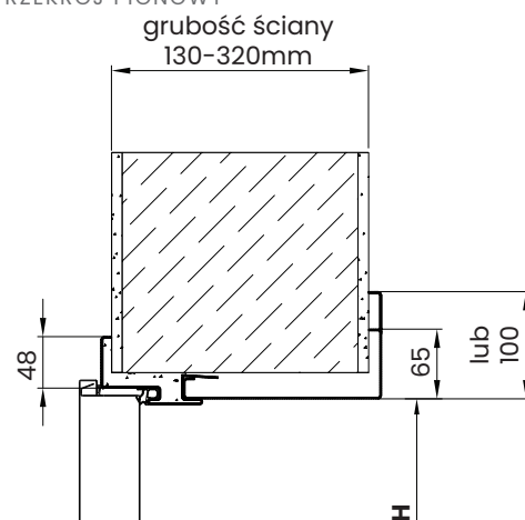
PRZEKRÓJ PIONOWY
