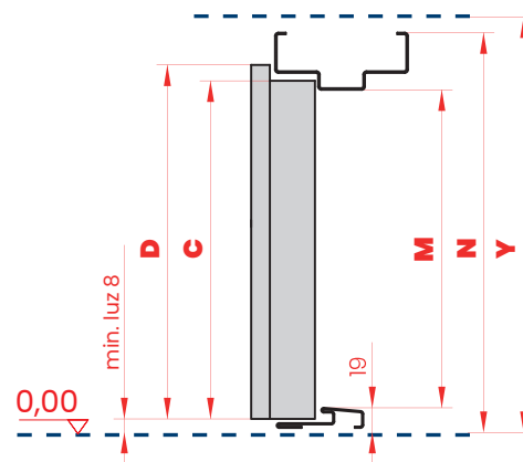
PRZEKRÓJ PIONOWY
