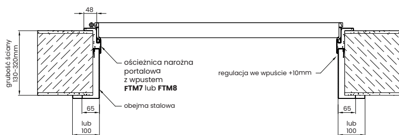
PRZEKRÓJ POZIOMY
