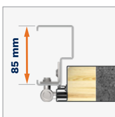
Ościeżnica stalowa FB
