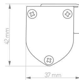
Rynna górna wraz z uchwytem montażowym
