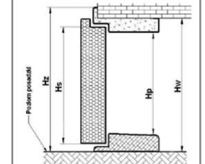
Rysunek poglądowy dla ościeżnic drzwi i progów dla: FN, FT SL
