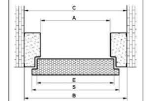
Rysunek poglądowy dla ościeżnic FC, FC SL, FD, FR, FR SL, FA SL
