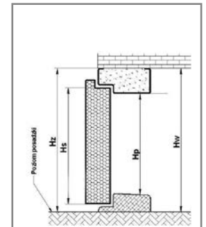
Rysunek poglądowy dla ościeżnic drzwi i progów dla: FD, FC, FC SL, FR, FR SL, FA SL
