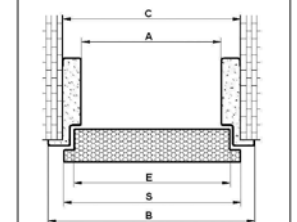
Rysunek poglądowy dla ościeżnic FN, FT SL
